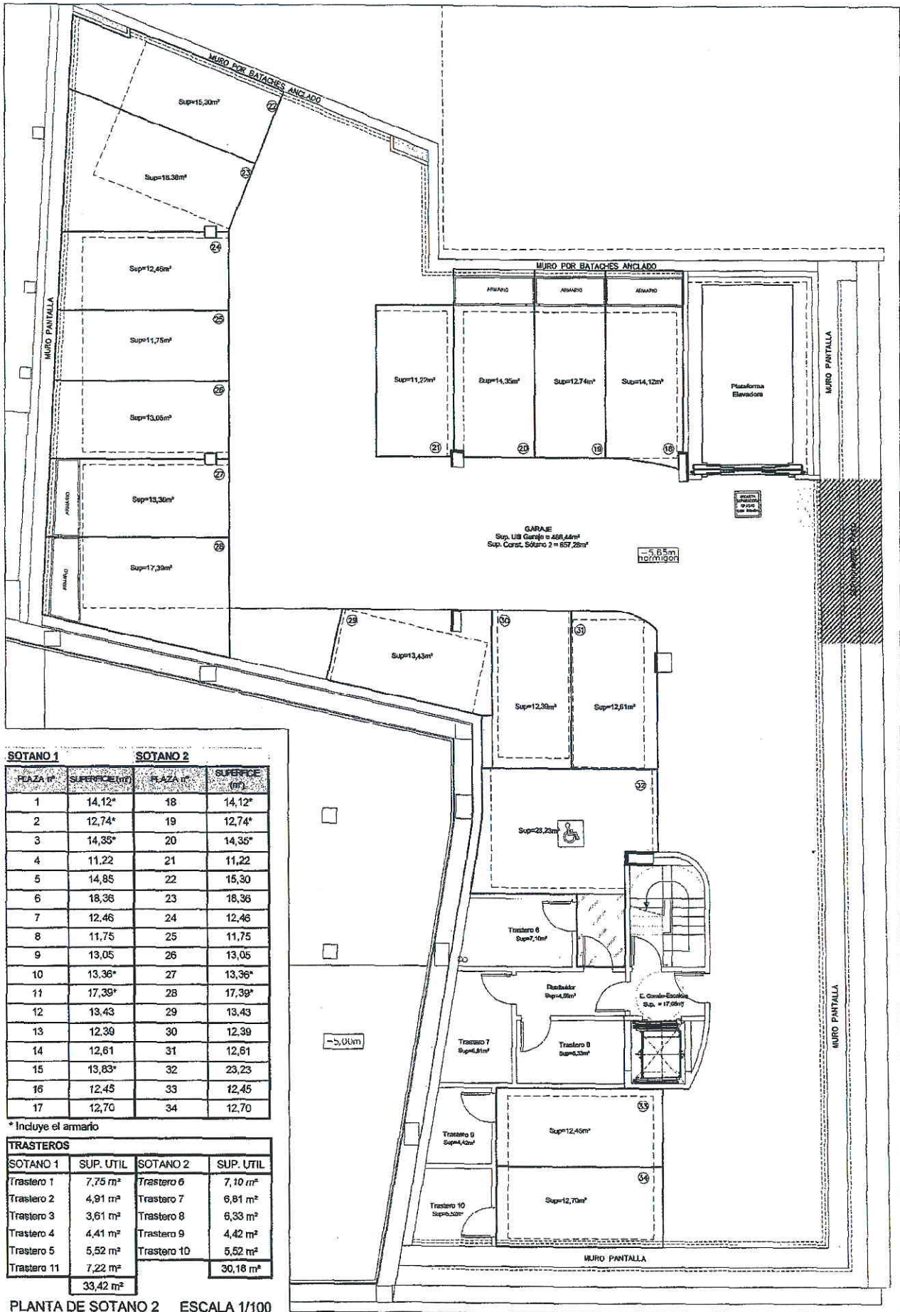
PLANTA DE SOTANO 2 ESCALA 1/100
